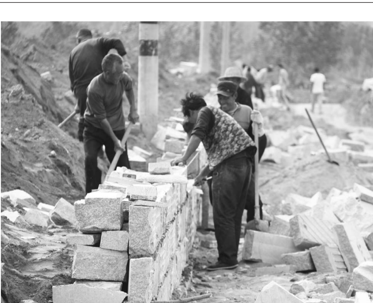
□孙涛 李丹 报道 近期，被列为国家水土保持重点建设工程的我县北山项目区高峪河小流域一期治理工程现场干劲火热朝天，施工人员正在争分夺秒的工作，努力在规定的节点完成施工任务。 该流域计划治理面积17.10km 2 ，主要采用工程、植物和封禁三大措施相结合的方法进行治理。项目总投资857.07万元，建设完成后，可年增蓄水保水量80.18万立方米、保土拦沙量2.29万吨，林草覆盖率可提高到18.99%，年均可增加收入867.93万元，工程效益显著。 图为施工人员正在建设高标准堰坝。
